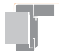
Détail: modèle à châssis affleurant design S (affleuré)
