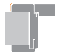
Détail: port affleurées design F avec contre-battu
