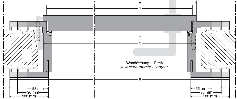
Querschnitt flächenbündig Section transversale à affleurement
