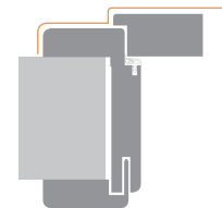
Détail: modèle à feuillure (standard)
